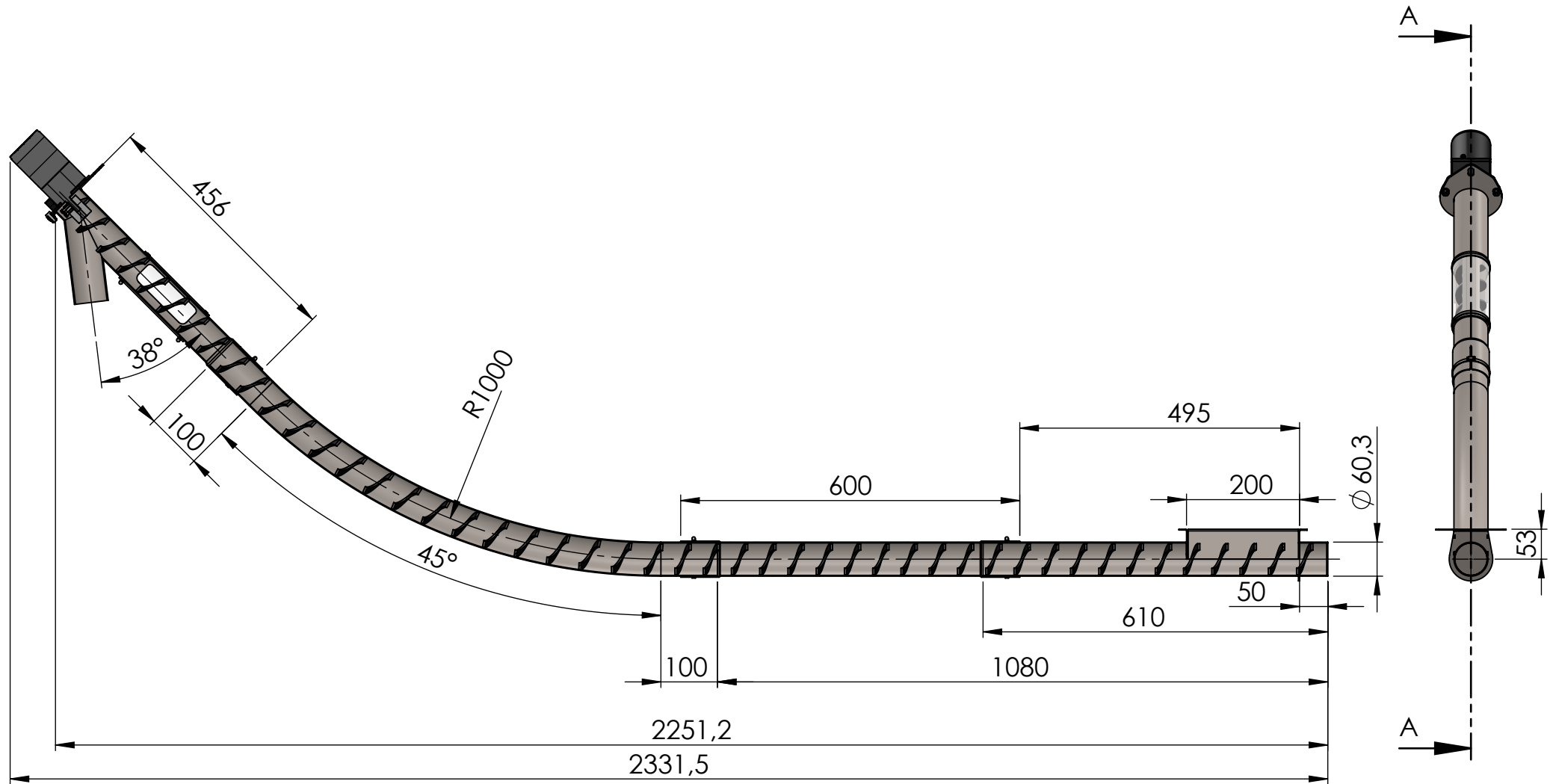
PRZEKRÓJ A-A
